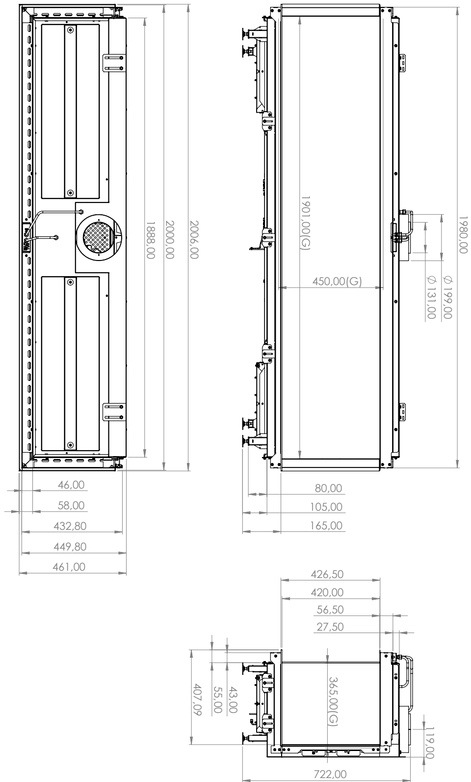
Figura I.3 - Disegno quotato Summum 190 3S
