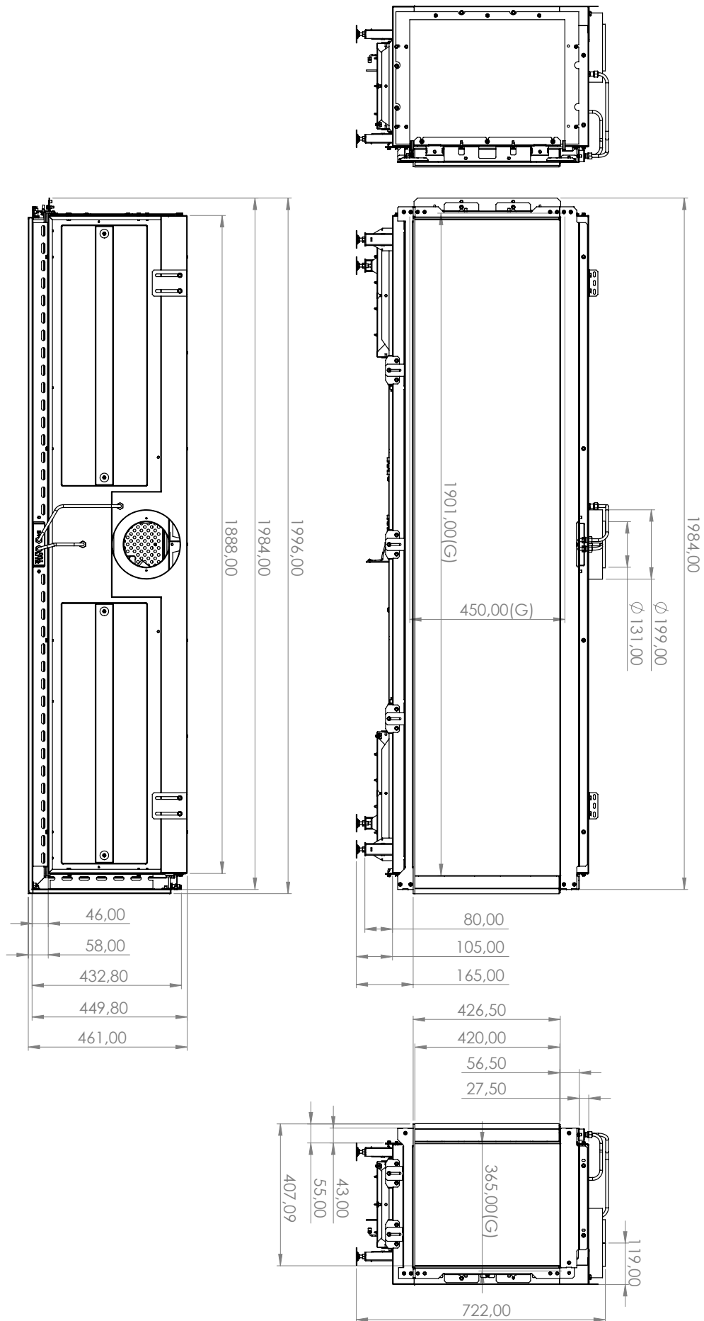
Figura I.2 - Disegno quotato Summum 190 C
