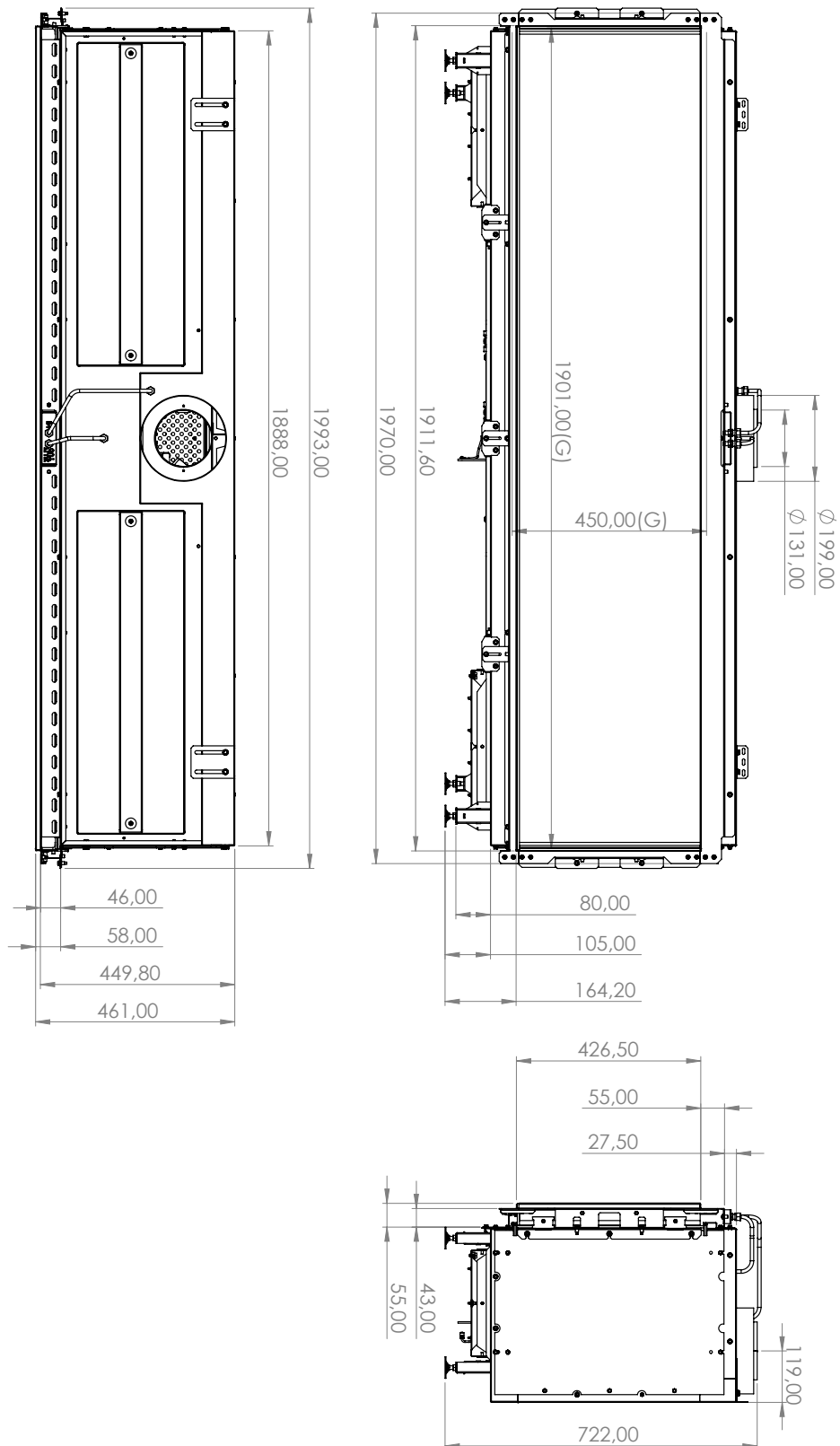
Figura I.1 - Disegno quotato Summum 190 F
