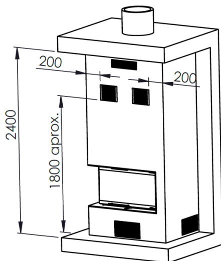
Figura n°10 - Schema esterno del rivestimento
