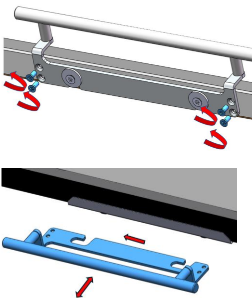
Figura n°44 - Estrazione delle viti e utilizzo come "maniglia fredda" per la maniglia
