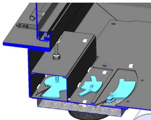
Figura n°47 - Accesso ai registri di entrata dell'aria
