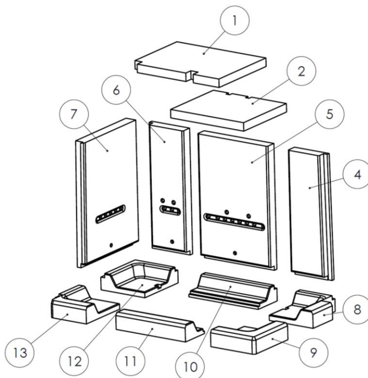
Figura nº52 - Pezzi principali vermi IZARO 80 CLD
