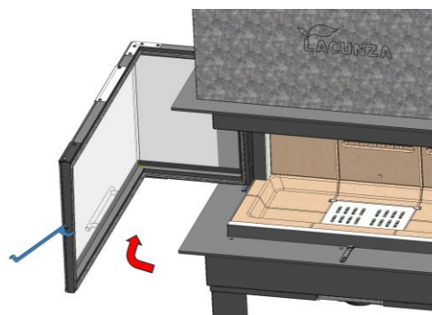
Figura n°43 - Porta aperta orizzontalmente
