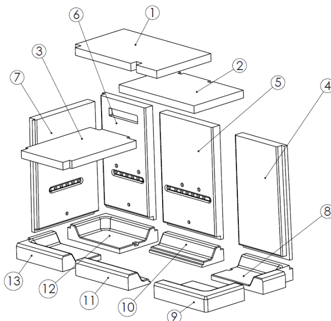
Figura nº53 - Pezzi principali vermi IZARO 100 CLD
