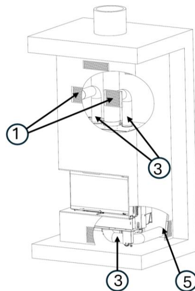
Figura n°16 - Immagine descrittiva dell'opzione D
