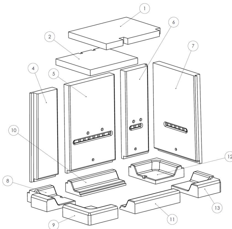
Figura nº49 - Vista explosa vermiculite IZARO 80 CLI
