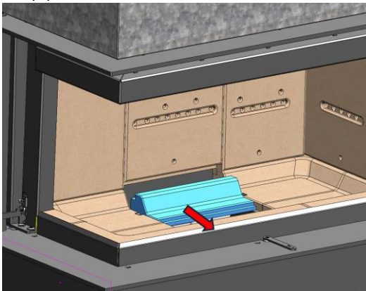
c- Rimuovere la base centrale posteriore (10) portandola in avanti
