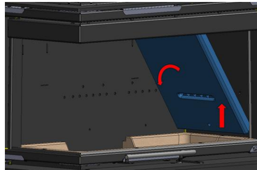
g- Rimuovere la piastra laterale posteriore sollevandola e lasciandola poi ricadere verso l'interno.
