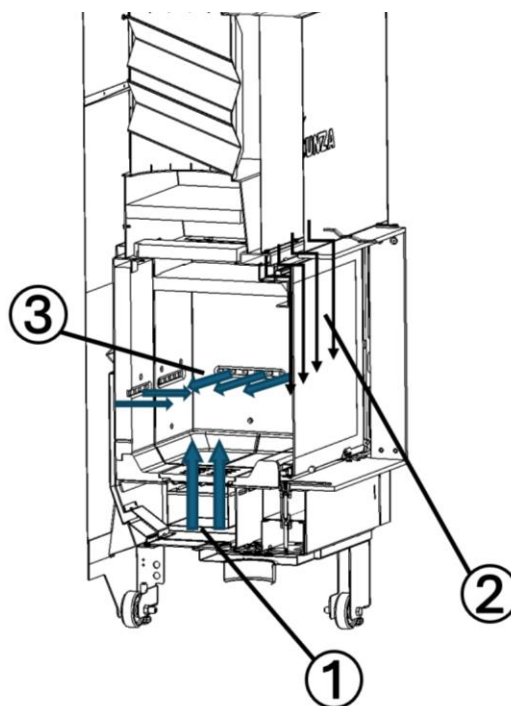
Figura n°32 - Ingresso d'aria comburente
