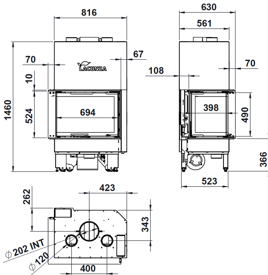
Figura nº1 - Dimensioni in mm dell'apparecchio IZARO 80 CLI
