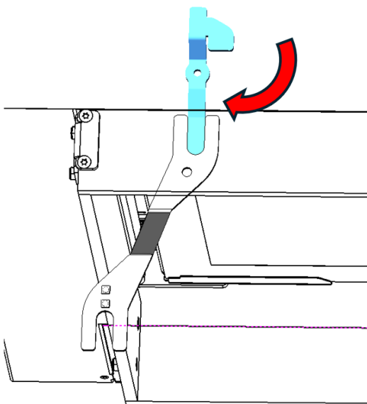
Figura n°41 - Girare la leva in alto a sinistra di 90° in senso orario
