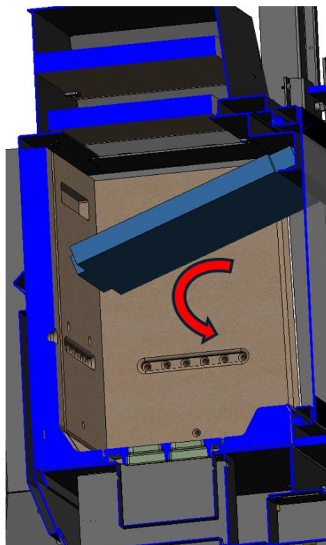
Figura n°35 - Smontaggio del deflettore inferiore dell'Izaro 100 CLI
