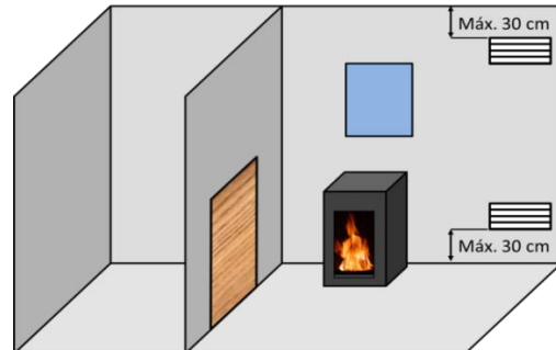
Figura n°6 - Schema orientativo per griglie di ventilazione
