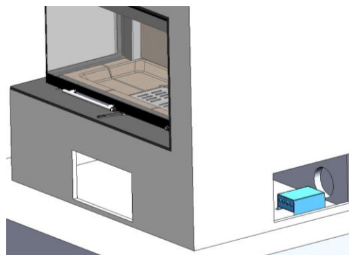
Figura n°23 - Posizionamento del modulo di potenza davanti alla griglia di ventilazione laterale
