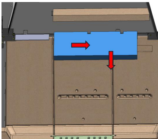
Figura n°36 - Smontaggio del deflettore medio Izaro 100 CLI
