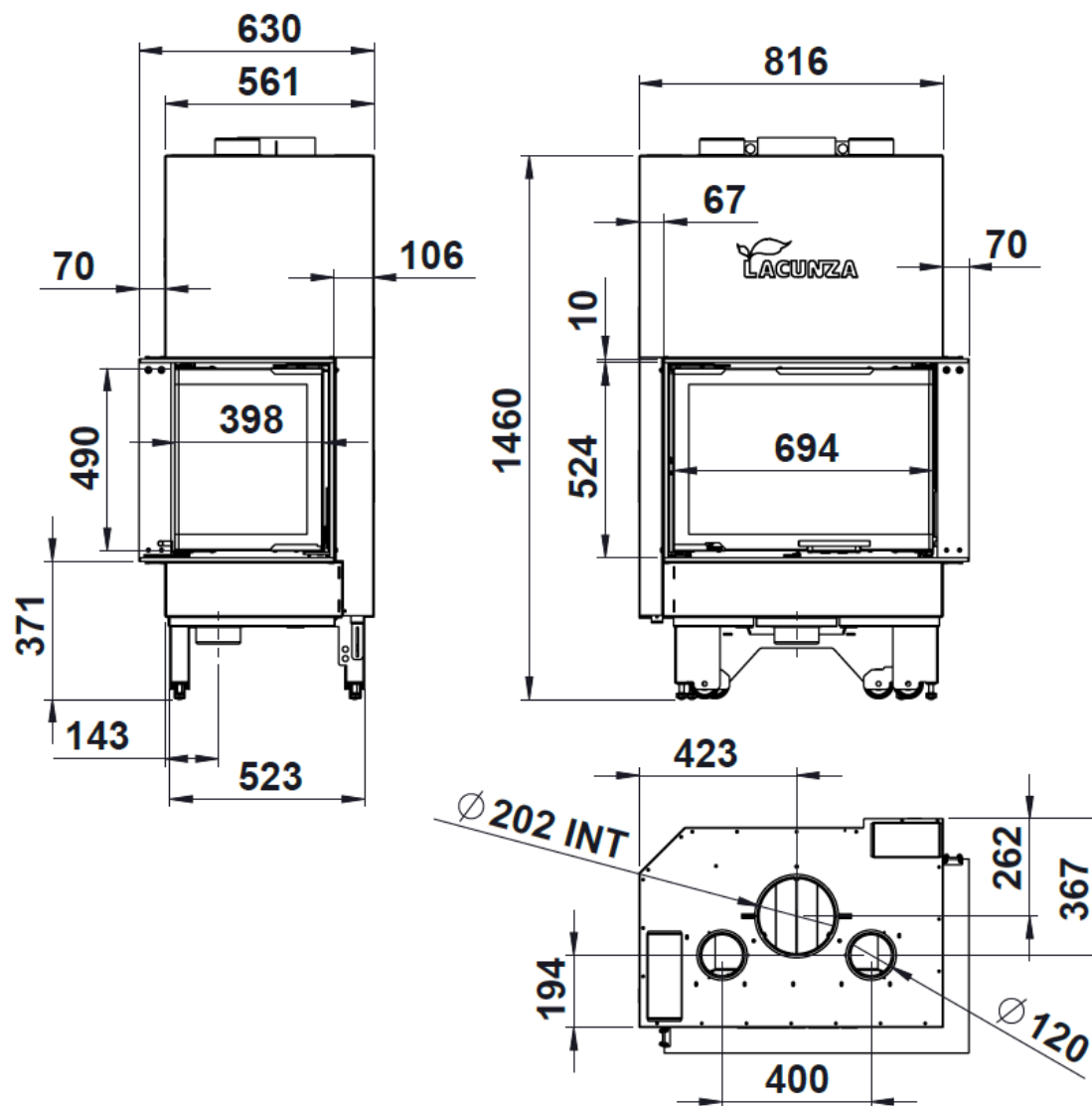
Figura n°3 - Dimensioni in mm dell'apparecchio IZARO 80 CLD
