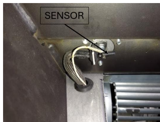
Figura n°24 - Posizione della sonda di temperatura (SENSOR) nell'uscita dell'aria della turbina
