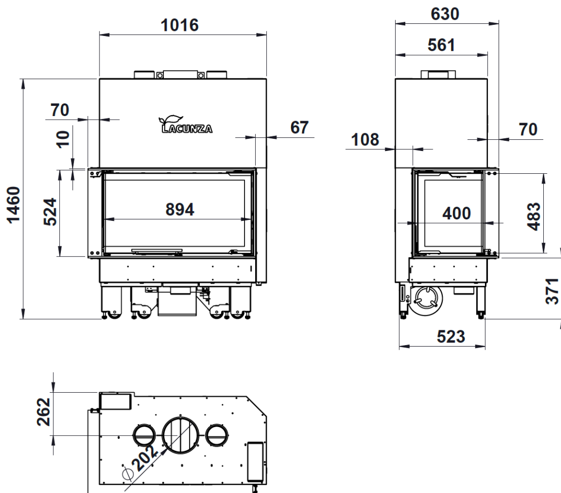
Figura n°2 - Dimensioni in mm dell'apparecchio IZARO 100 CLI
