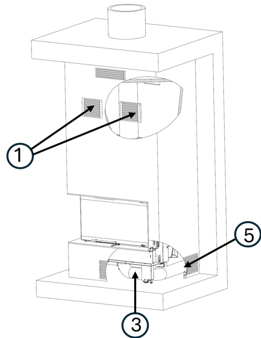
Figura n°15 - Immagine descrittiva dell'opzione C
