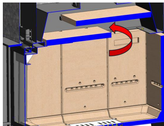
Figura n°31 - Rimozione del deflettore inferiore per ridurre l'intonaco IZARO 100 CLI.
