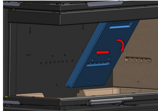
f- Rimuovere la piastra posteriore destra (6) spostandola verso l'interno e lasciandola cadere in avanti.
