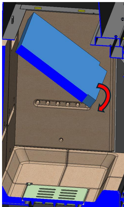
Figura n°37 - Smontaggio del deflettore superiore dell'Izaro 100 CLI
