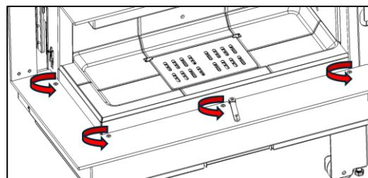
Figura n°17 - Allentare le 8 viti, 4 superiori e 4 inferiori che fissano la cornice esterna
