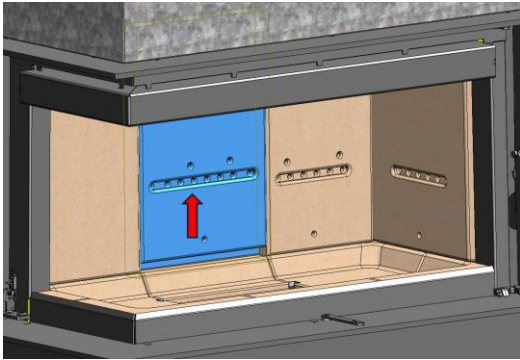
b- Sollevare la piastra posteriore centrale (5)
