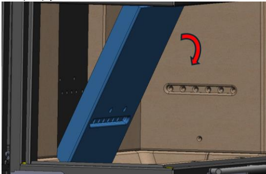
d- Rimuovere la piastra centrale posteriore (5) lasciandola cadere in avanti.
