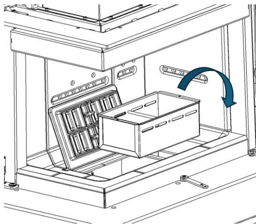
Figura n°33 - Estrazione del cassetto posacenere
