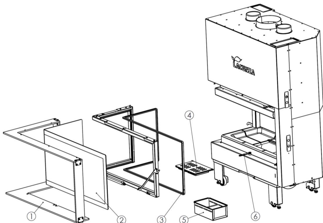
Figura nº48 - Pezzi principali Izaro 80-100 CLI
