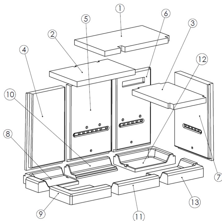
Figura nº50 - Pezzi principali vermi IZARO 100 CLI
