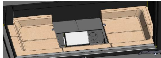
h- Rimuovere il resto delle basi in vermiculite (8), (9), (11), (12), (13).
