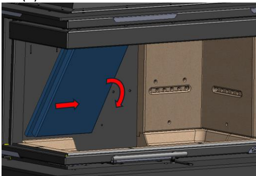
e- Rimuovere la piastra posteriore sinistra (4) spostandola verso l'interno e lasciandola cadere in avanti.
