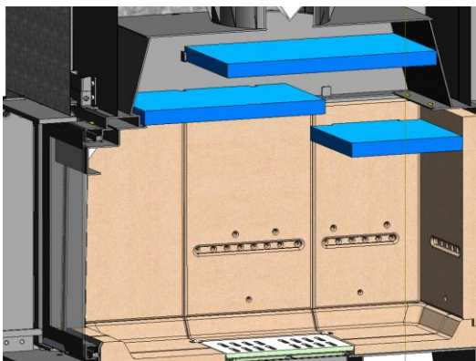
Figura n°34 - Vista in sezione dell'Izaro 100 CLI con i 3 deflettori posizionati
