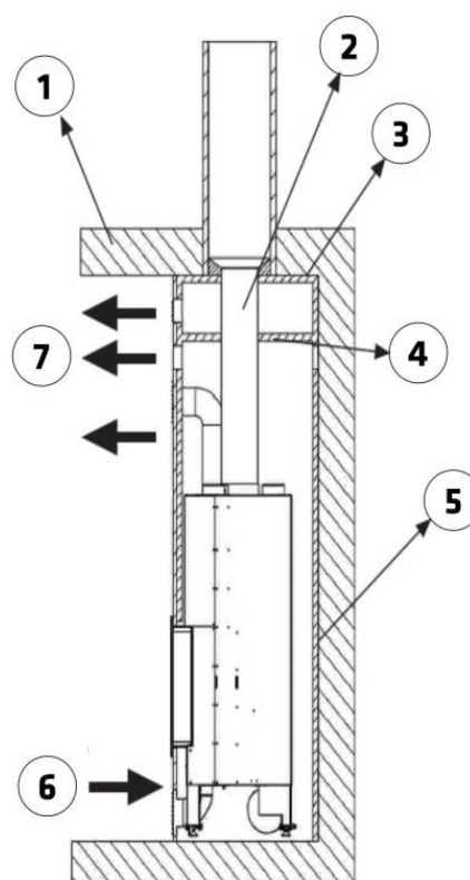
Figura n°9 - Schema interno del rivestimento
