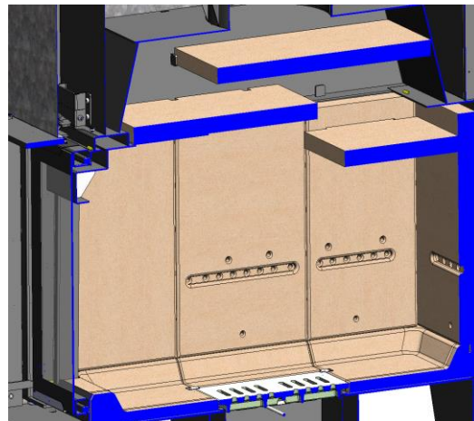
Figura n°30 - Posizione attuale dei deflettori IZARO 100 CLI
