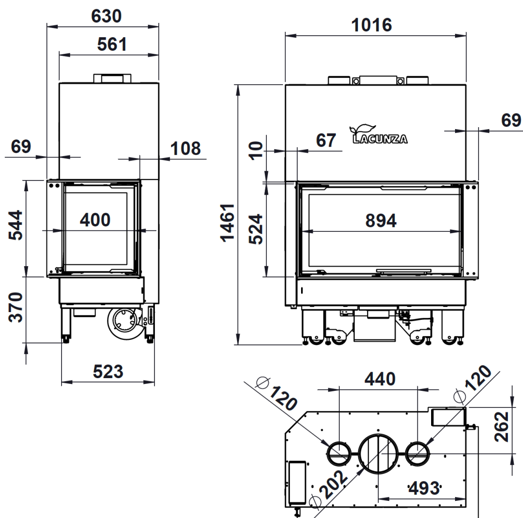
Figura n°4 - Dimensioni in mm dell'apparecchio IZARO 100 CLD
