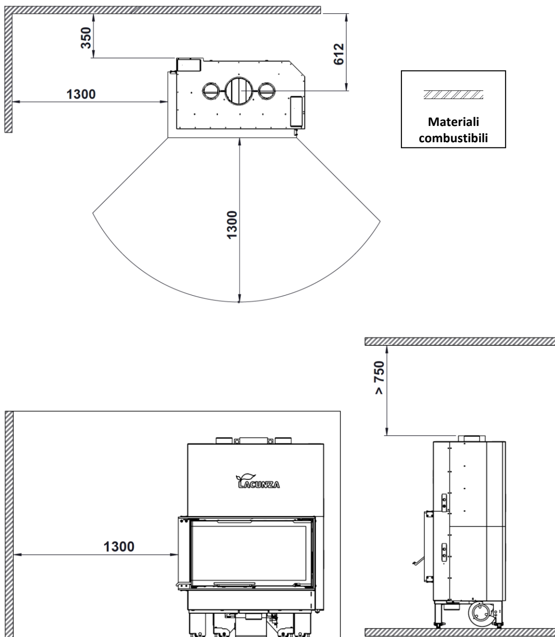
Figura n°5 - Distanze di sicurezza Izaro 80-100 CLI
