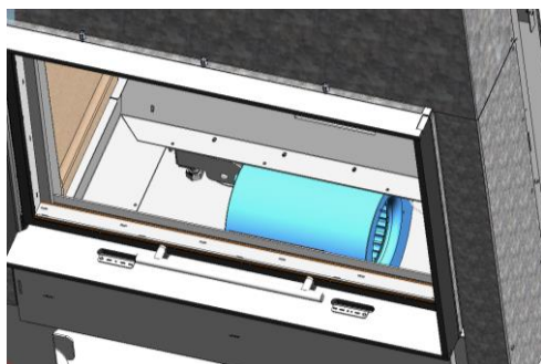
Figura n°46 - Accesso alla turbina attraverso l'interno del focolare
