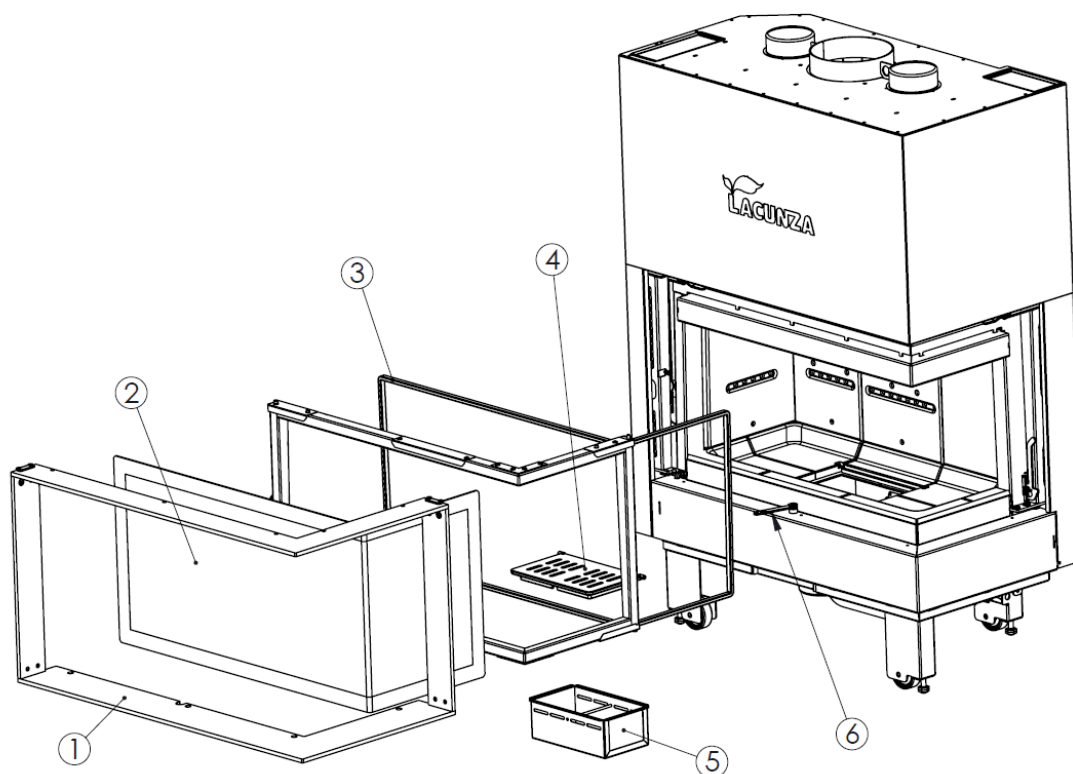
Figura nº51 - Pezzi principali Izaro 80-100 CLD
