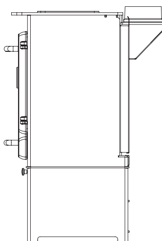
END ELEVATION
