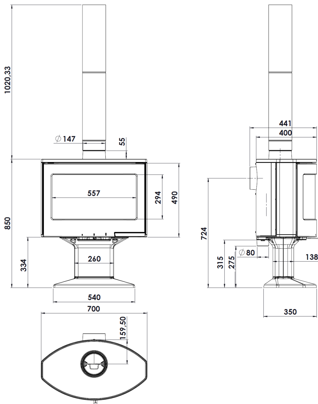
Figura n°1 - Dimensioni in mm dell'apparecchio Tarbes Star
